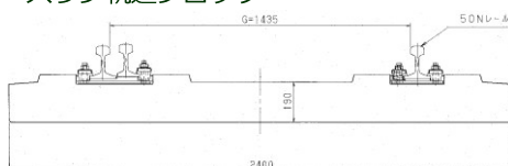
スラブ軌道ブロック
