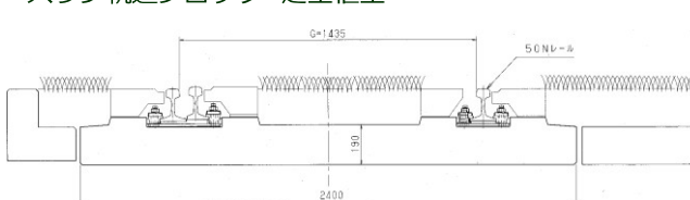
スラブ軌道ブロック 芝生植生
