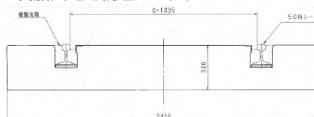
樹脂固定用軌道ブロック
