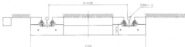
スラブ軌道ブロック 芝生植生
