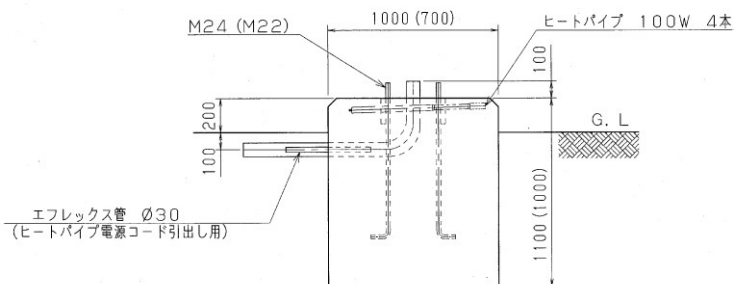
警報機（しや断機）基礎断面
