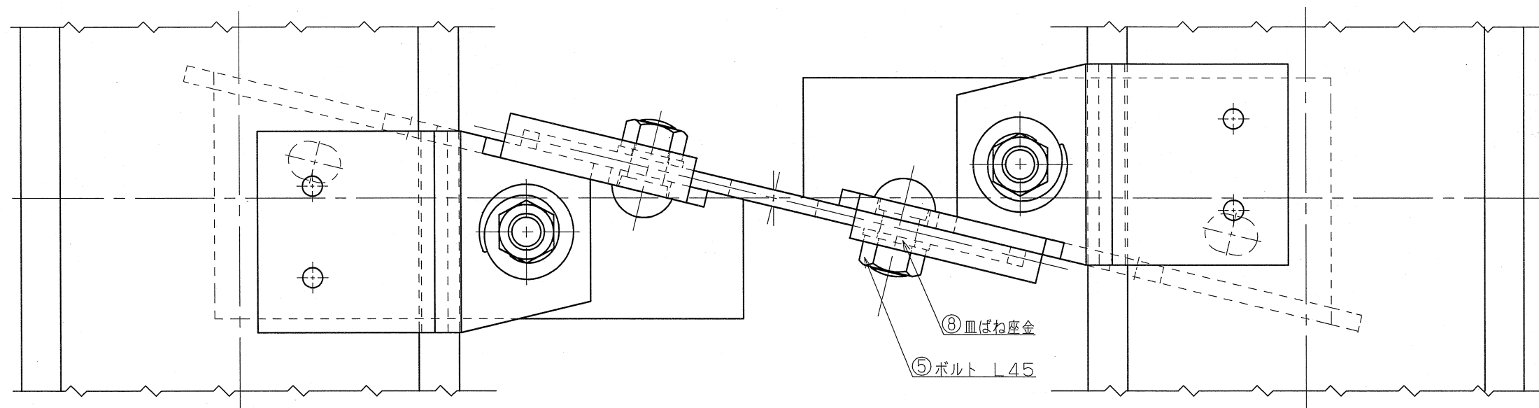
組立図 S=1/2
