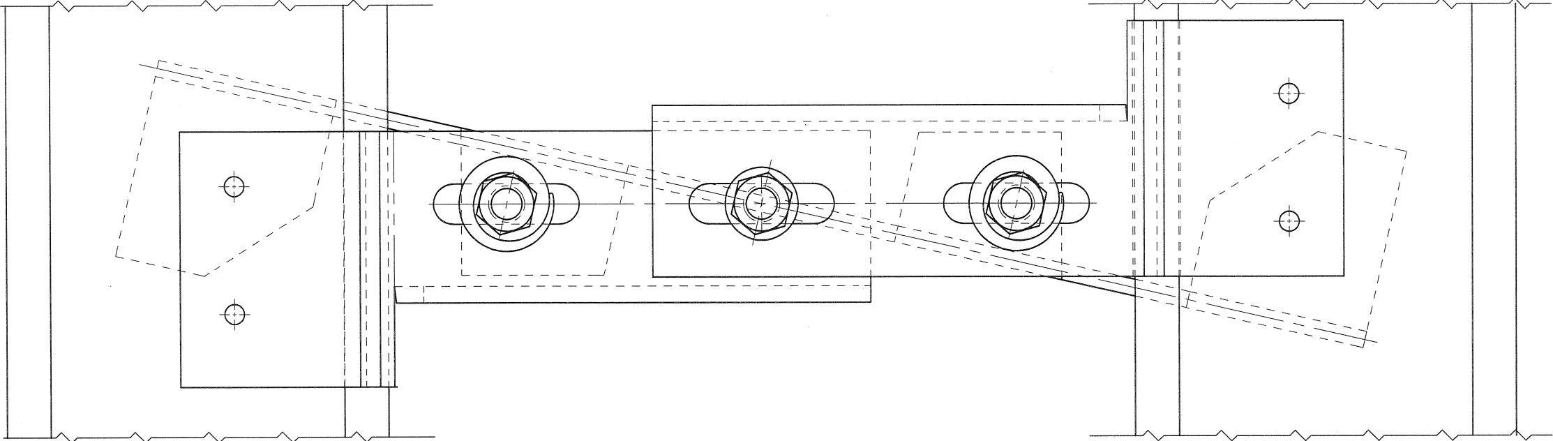
組立図 S=1/2
