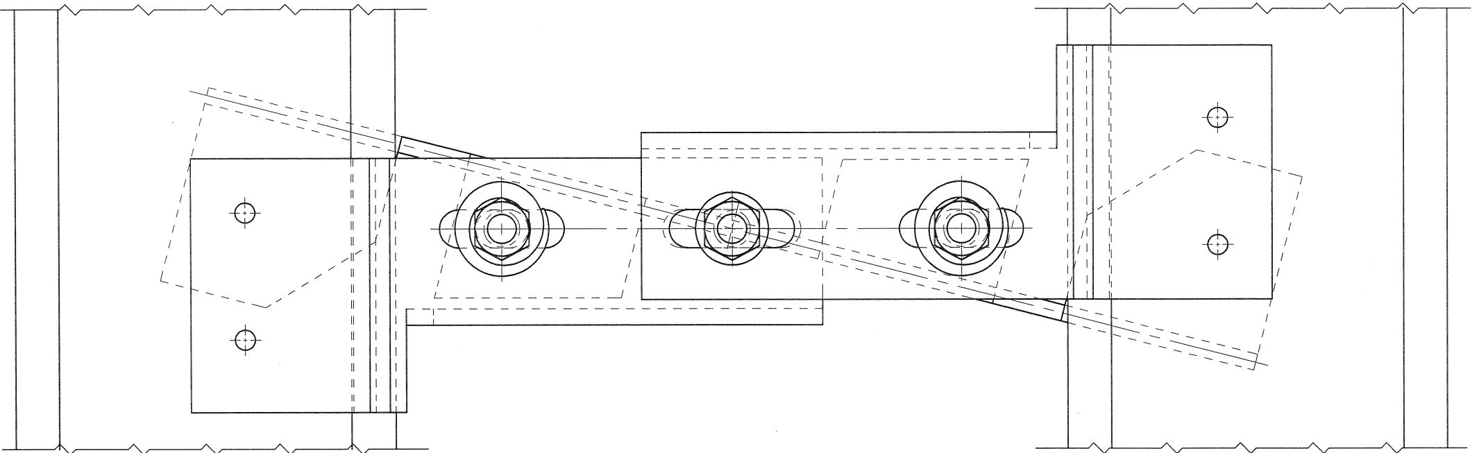
組立図 S=1/2
