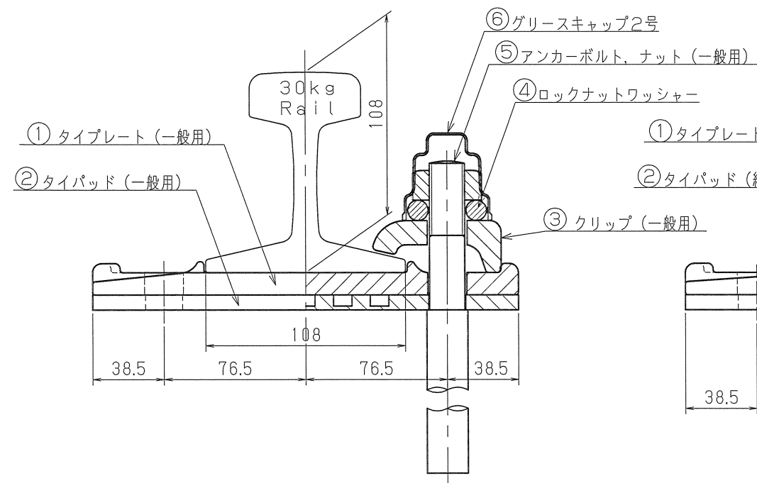
一般部締結図
