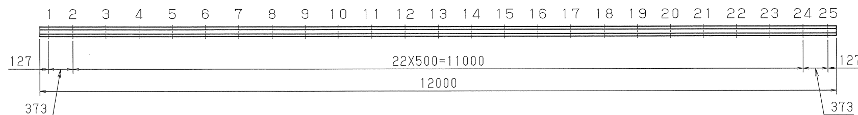
締結装置標準配列図
