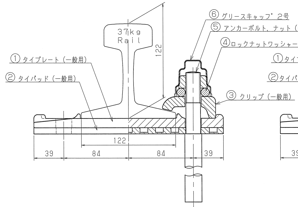
一般部締結図
