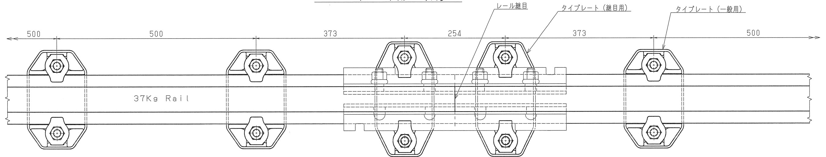
レール継目部附近取付図
