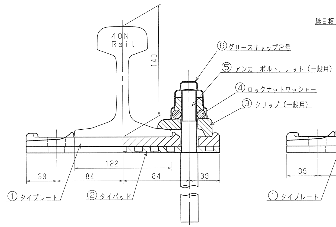
一般部締結図
