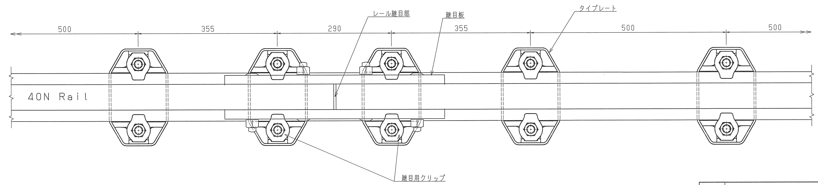
締結装置標準配列図
