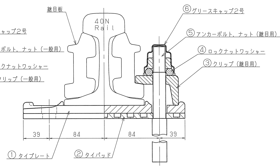
継目部締結図
