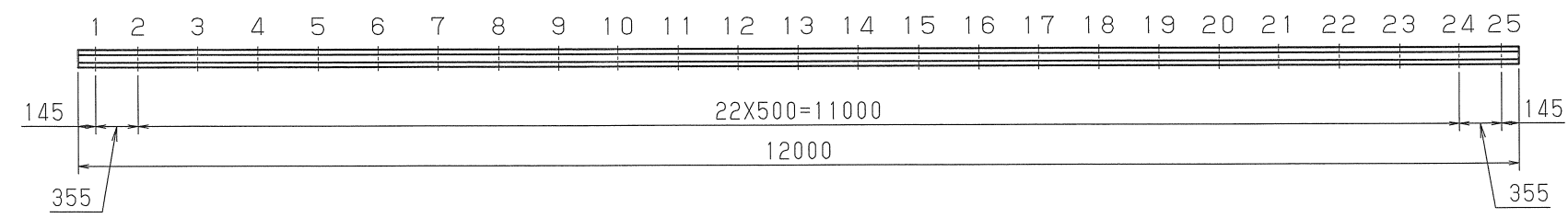
締結装置標準配列図
