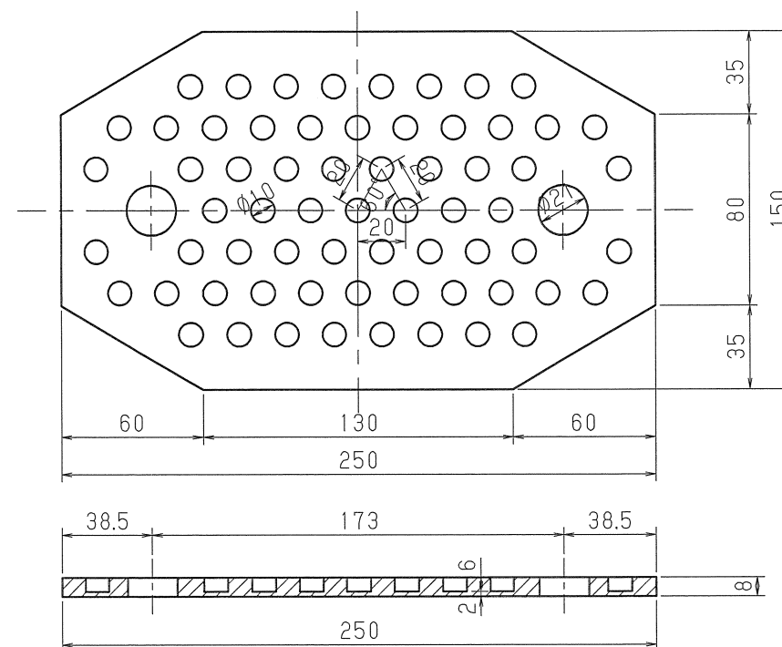
② タイパッド
