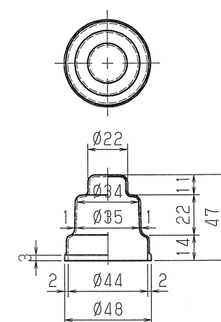
⑥ グリースキャップ 2号
