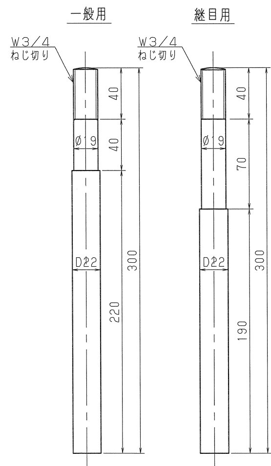
⑤ アンカーボルト, ナット
