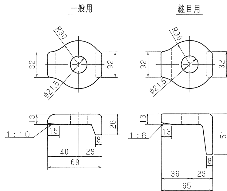
③ クリップ
