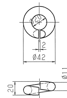
④ ロックナットワッシャー
