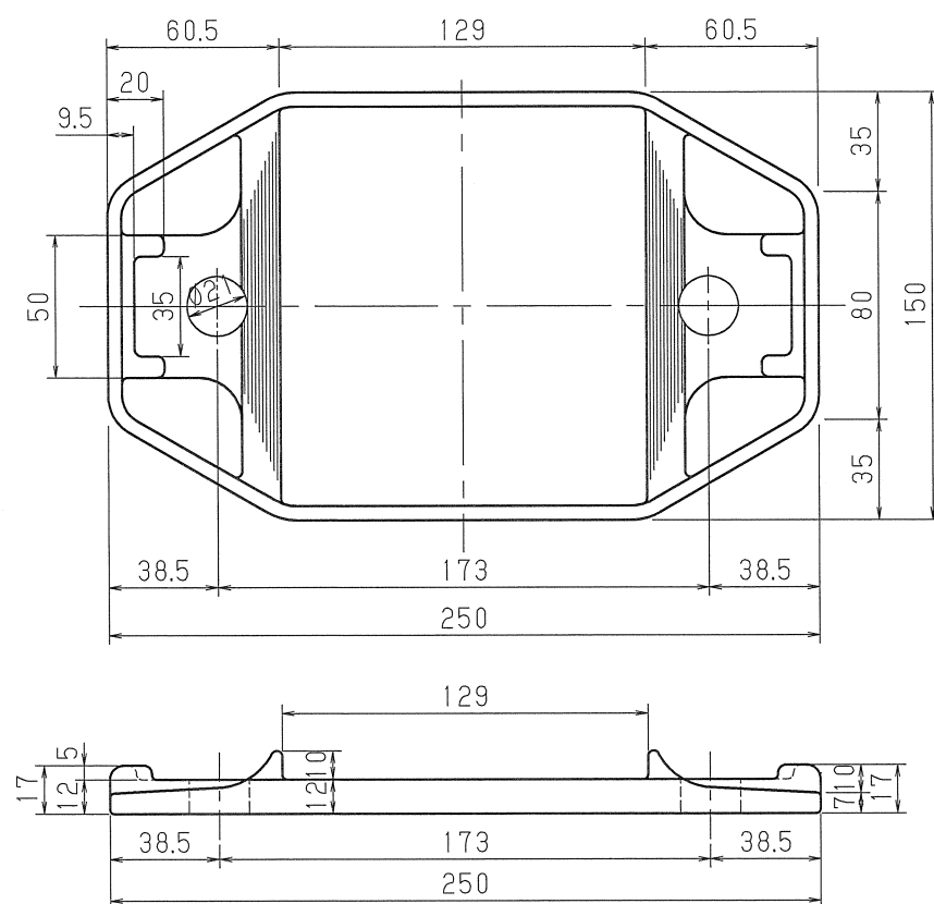
① タイプレート
