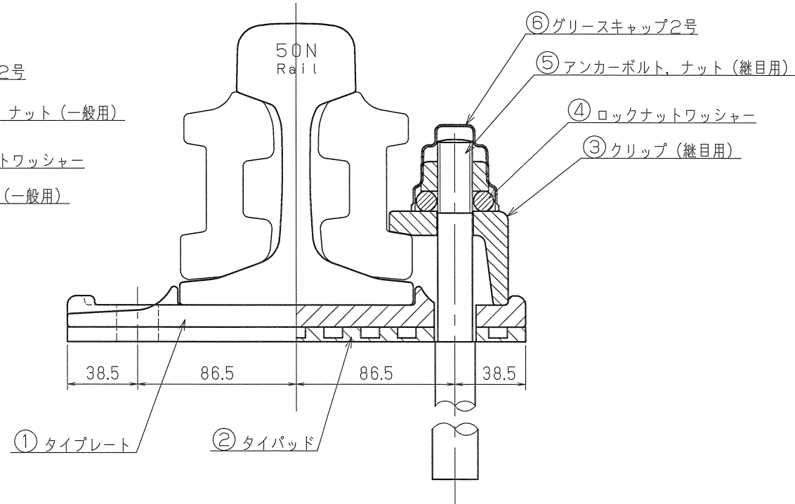
レール継目部附近取付図
