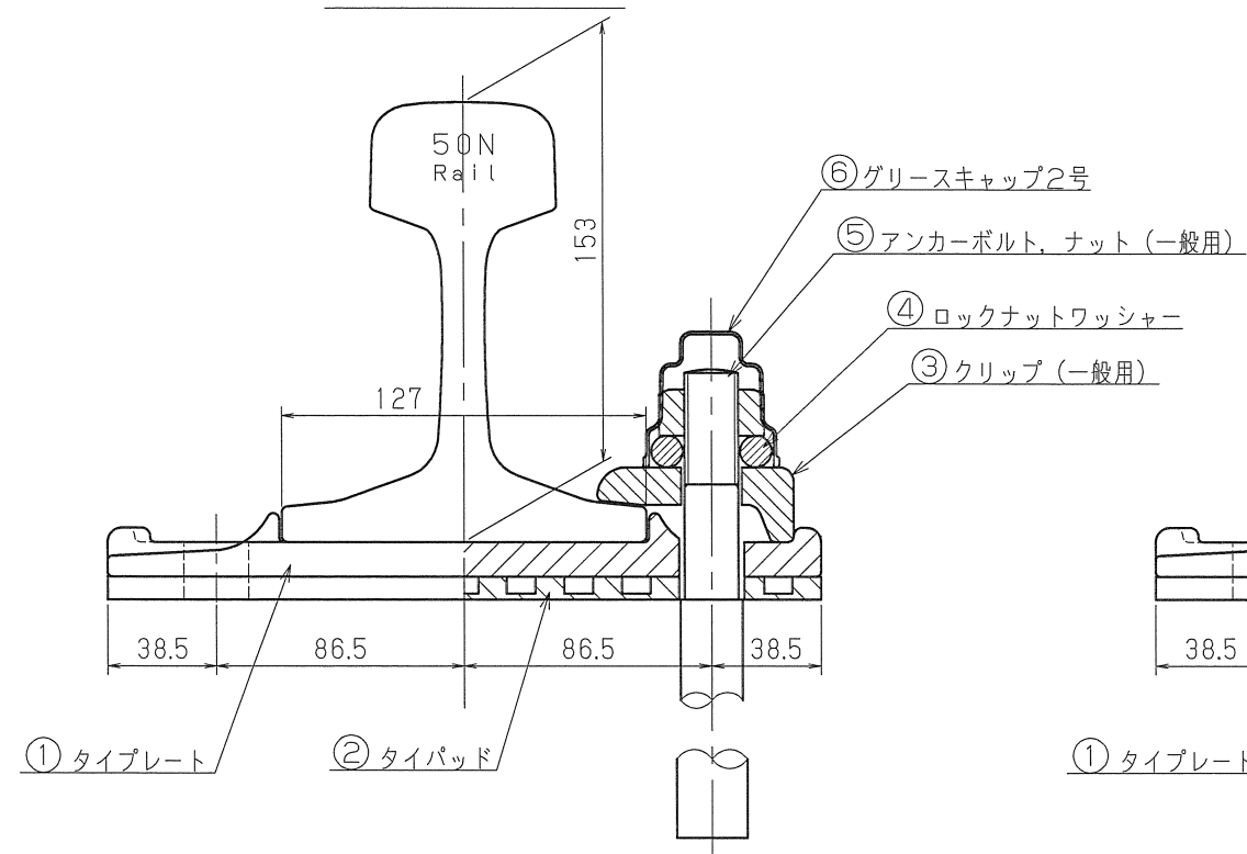
一般部締結図
