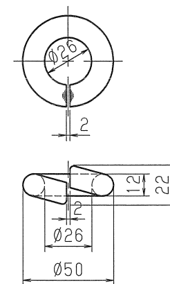
④ ロックナットワッシャー
