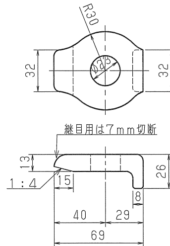
③ クリップ
