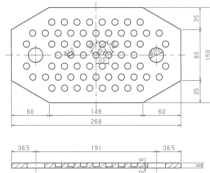
② タイパッド
