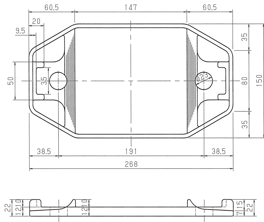
① タイプレート
