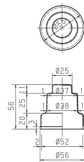
⑥ グリースキャップ 1号
