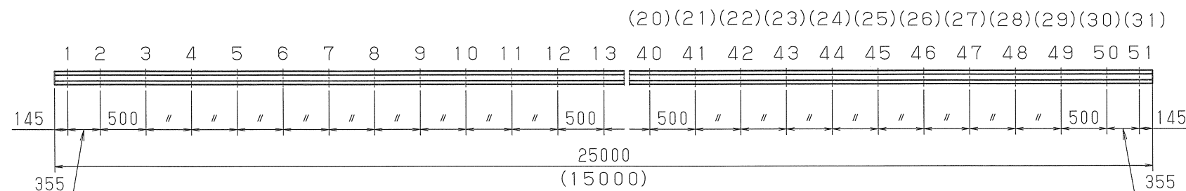
締結装置標準配列図
