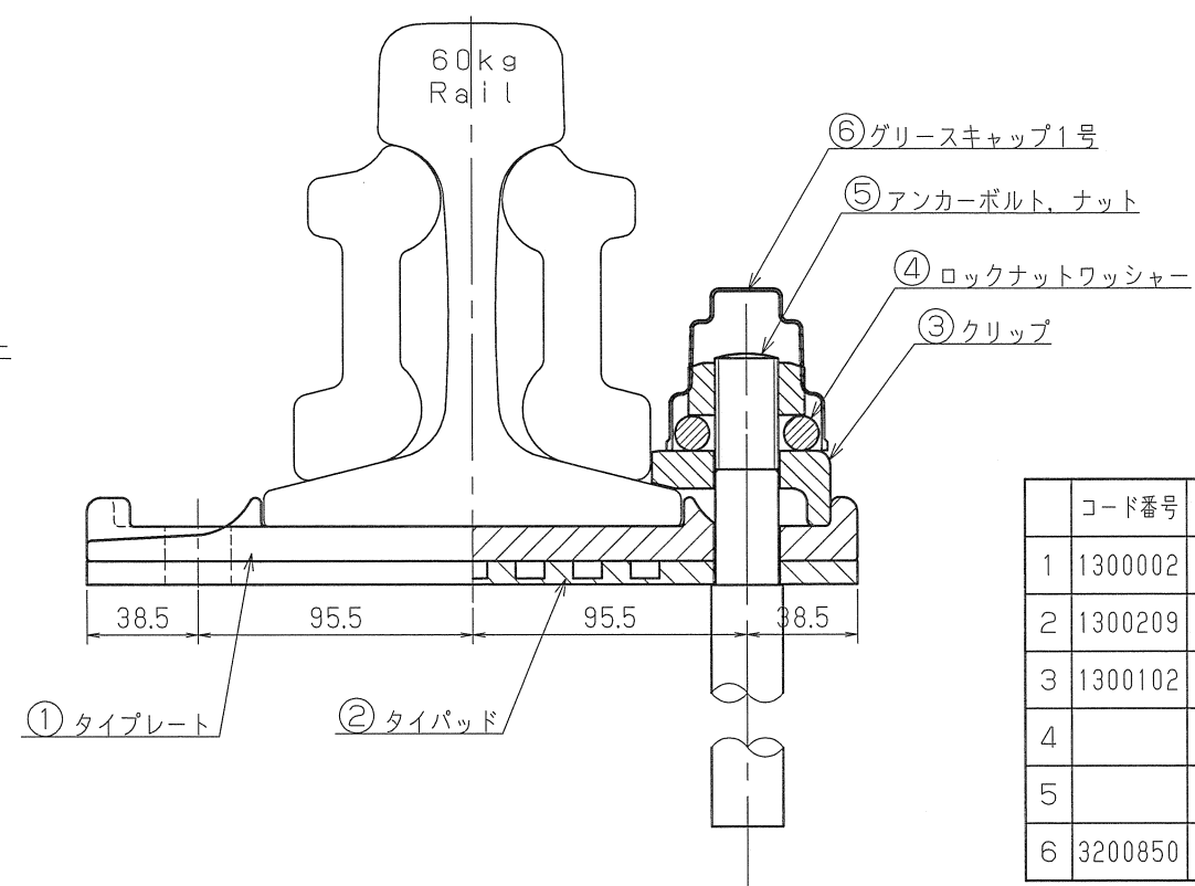
レール継目部附近取付図
