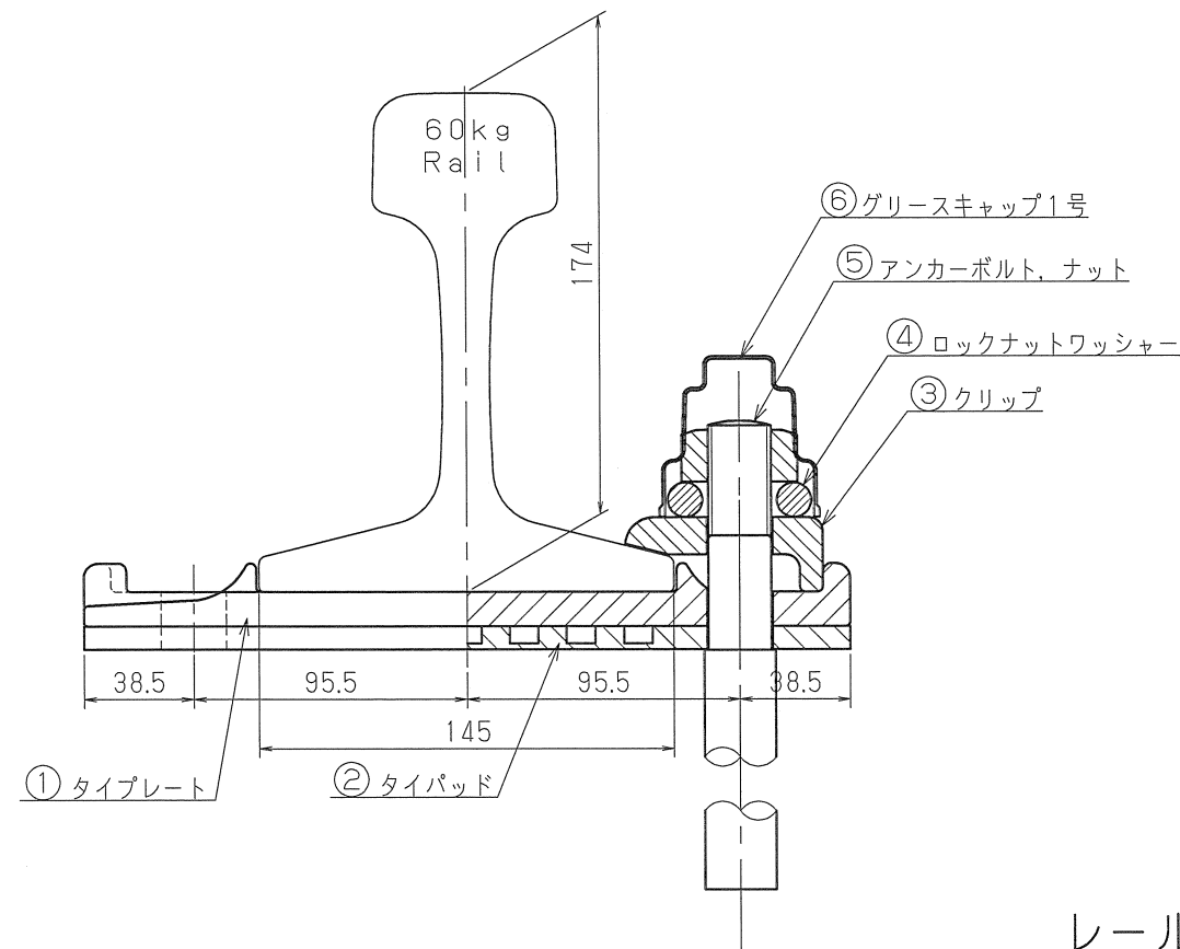
一般部締結図
