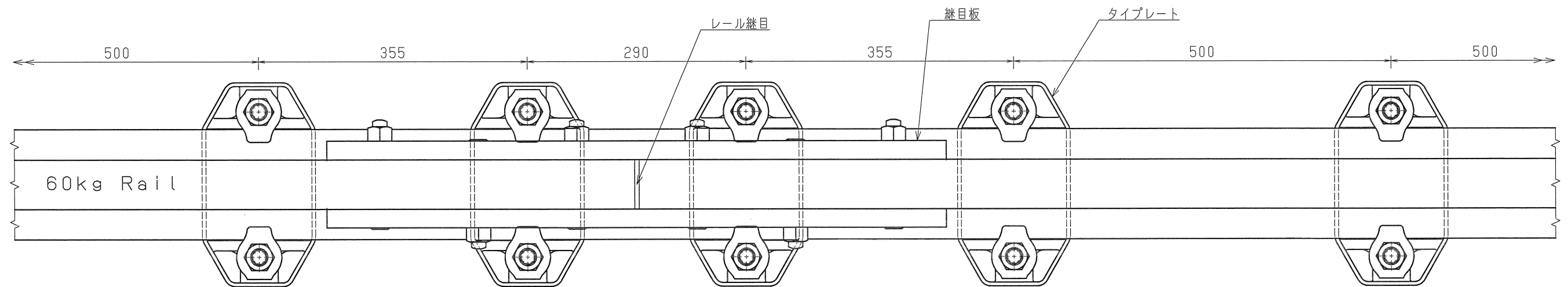
レール継目部附近取付図
