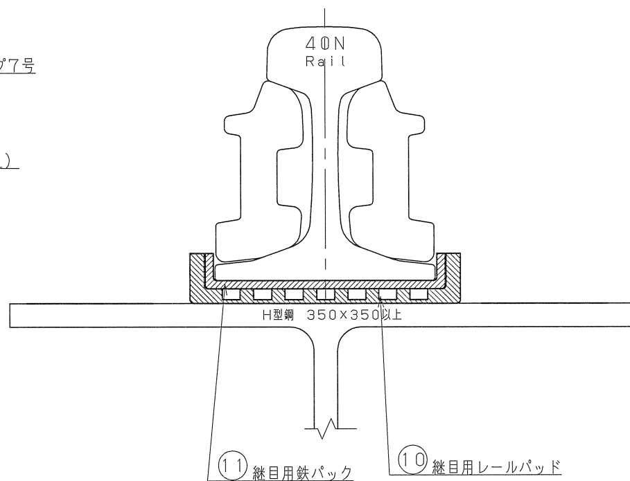
レール継目部附近取付図
