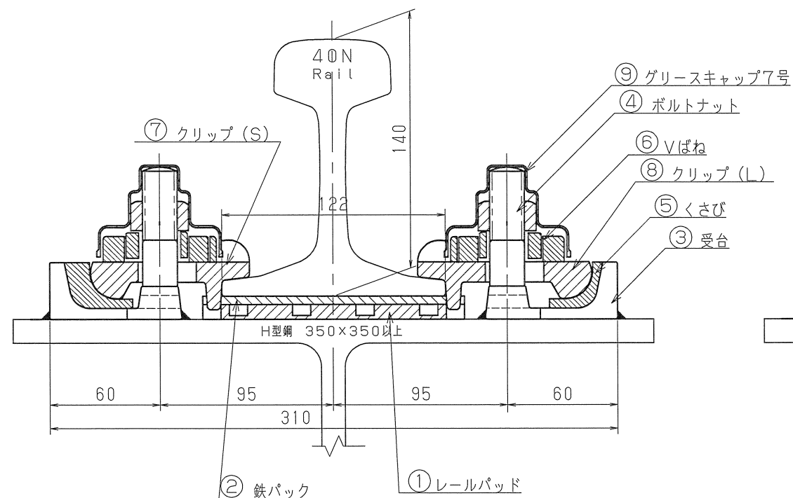
レール継目部附近取付図
