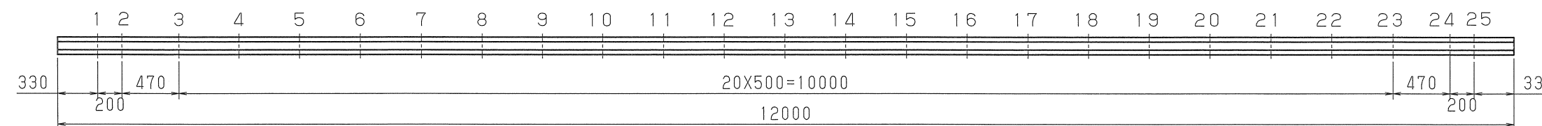
締結装置標準配列図
