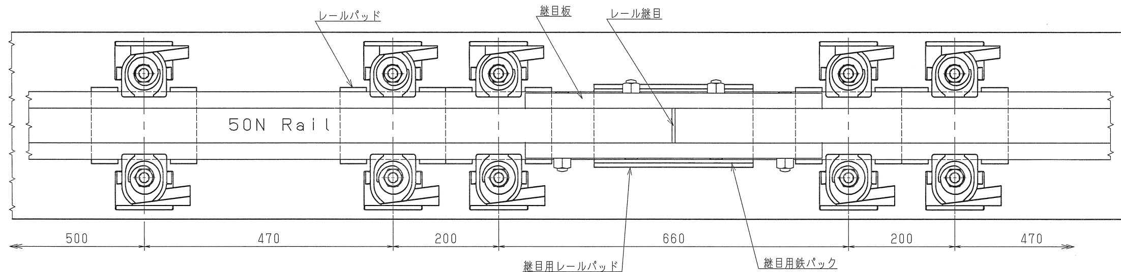
締結装置標準配列図
