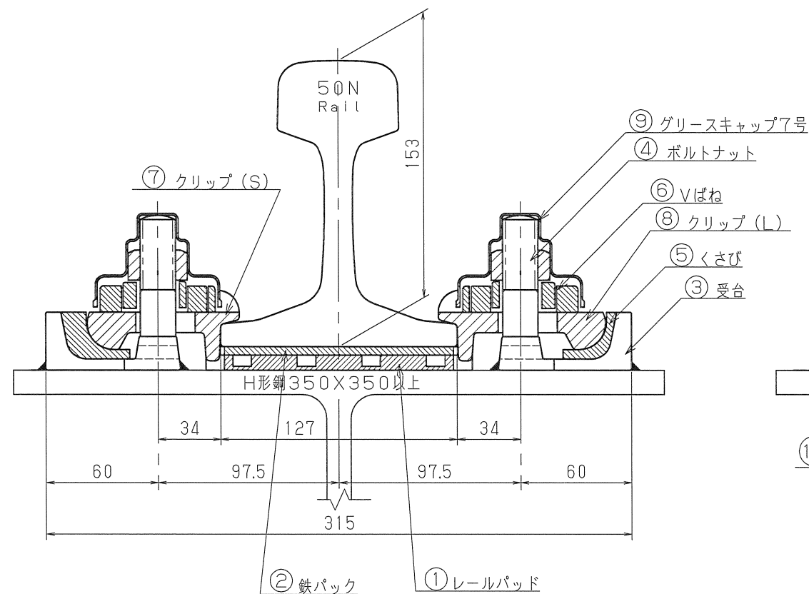
レール継目部附近取付図
