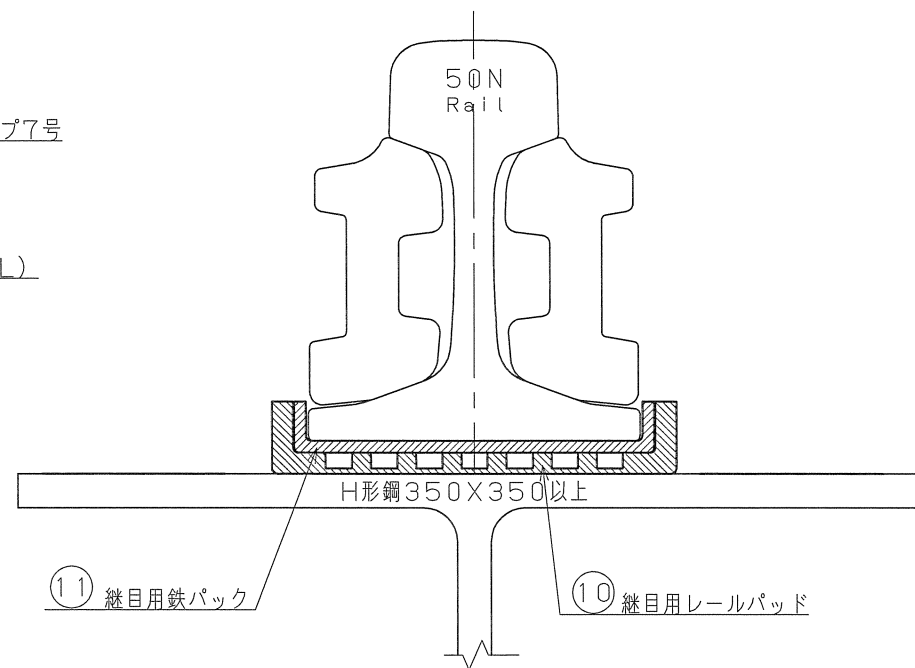
継目部締結図
