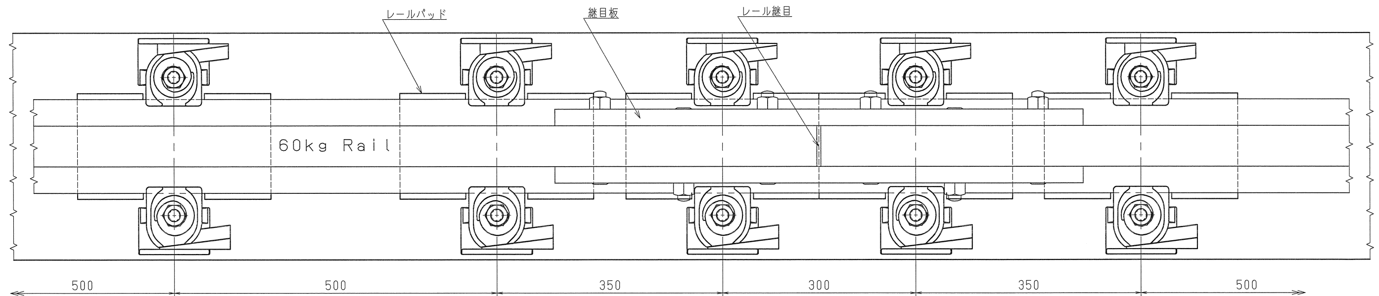
レール継目部附近取付図
