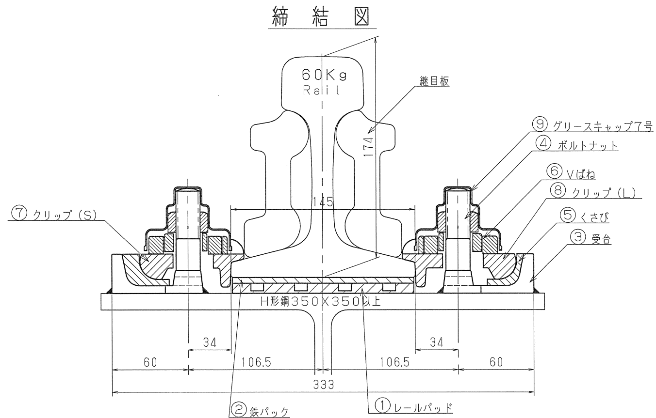
レール継目部附近取付図
