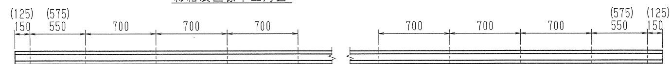
締結装置標準配列図 ( ) 寸法は50PS, 37, 30
