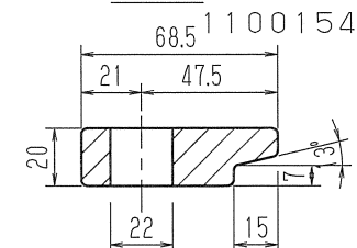
継目板加工図
