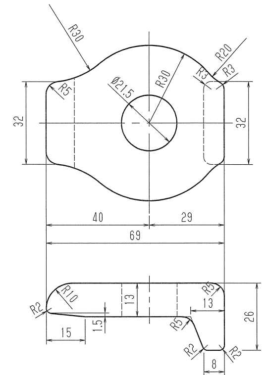
② クリップ
