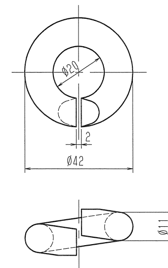
③ ロックナットワッシャー
