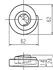
⑦ V ばね
