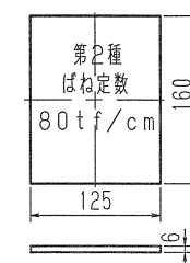
⑫ レールパッド
