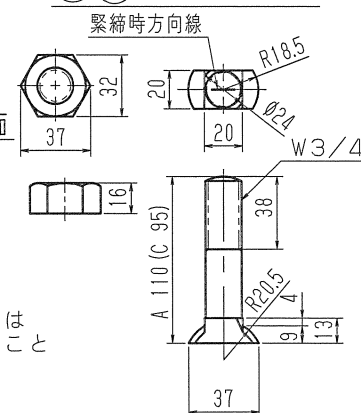
⑤⑥ ボルトナットA, C
