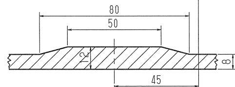
D-D' 断面
