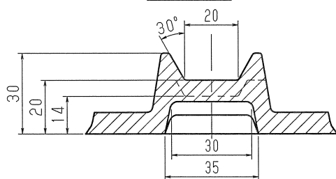
A-A' 断面
