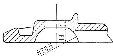
B-B' 断面
