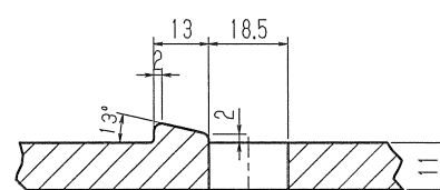
D-D' 断面
