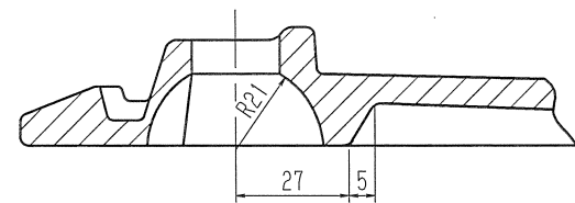
B-B' 断面
