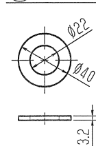
⑫ 平座金
