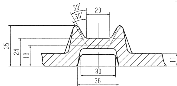
C-C' 断面
