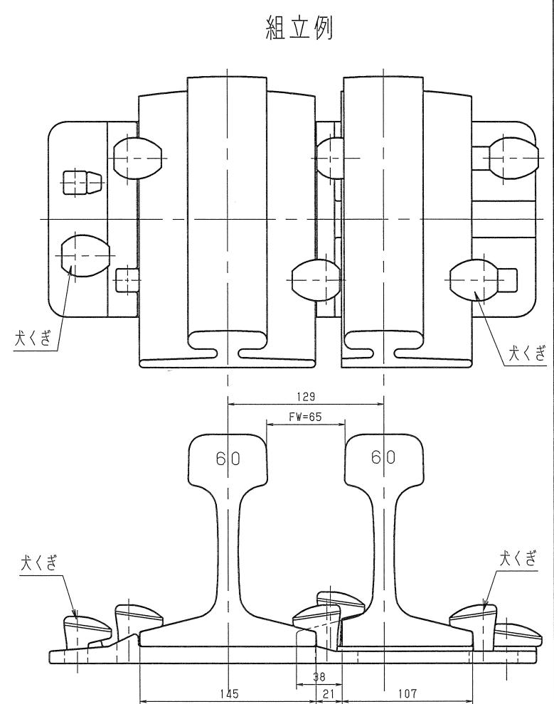
犬くぎはタイプレート用犬くぎ使用 ガードレール標準底部切欠量 38mm
